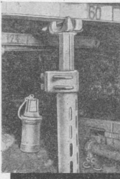
GHH-Strebausbau in Stahlleichtbauweise
