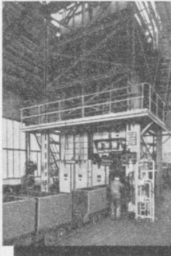
GHH-Schacht-Wetterschleuse
