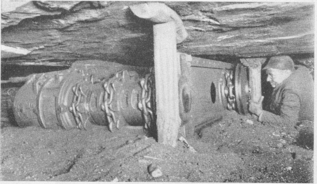
Abb. 4 Dreifaches Kettenband
