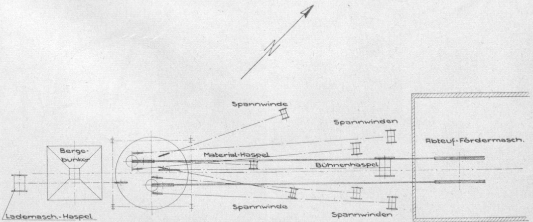
Abb. 2 Übersicht der Abteufeinrichtung
