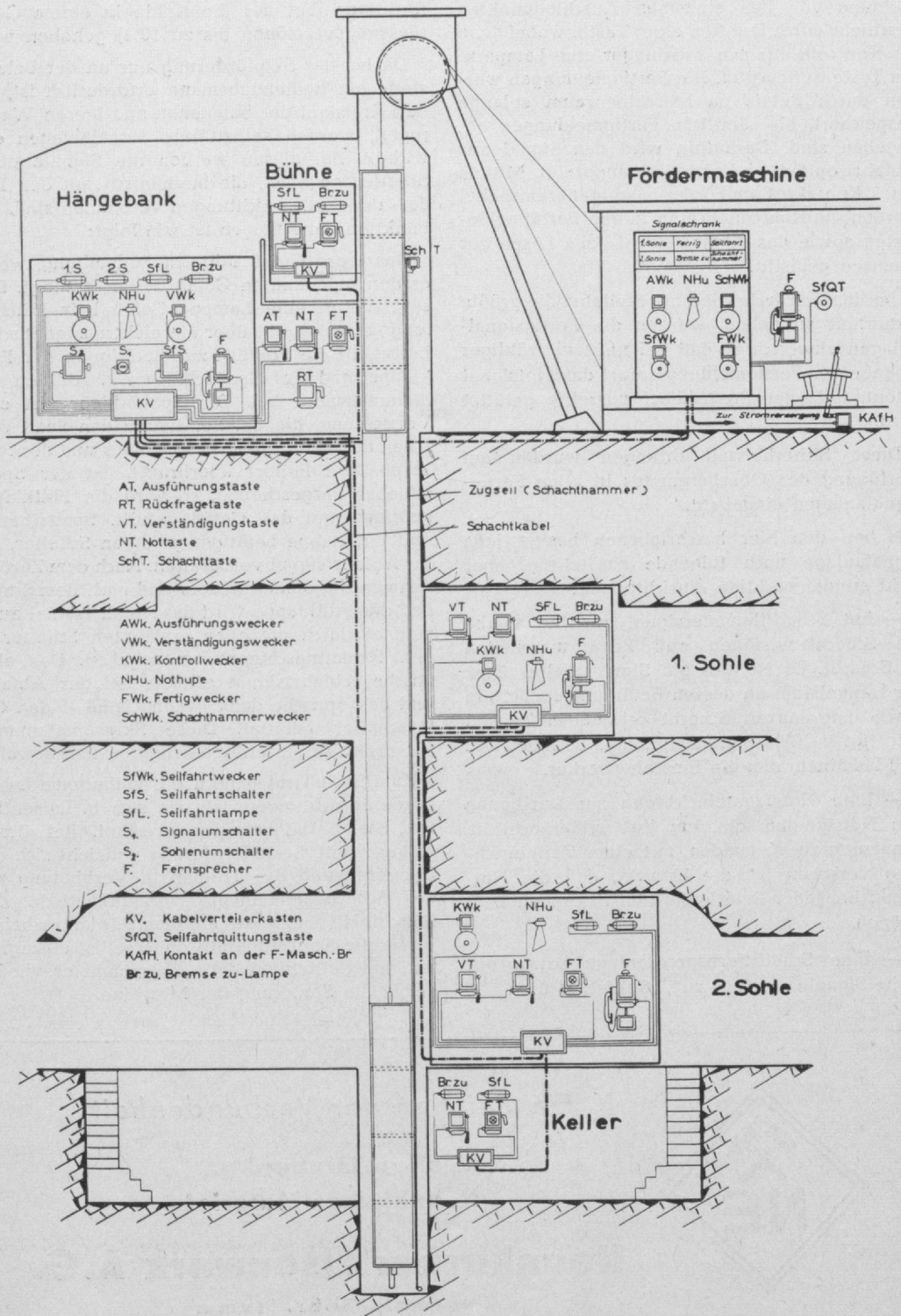
Schematische Darstellung einer Schachtsignalanlage für einen Hauptförderschacht
