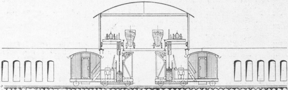
Doppel-Stampf-Anlage D.-R.-P. mit feststehender Füllstation.
