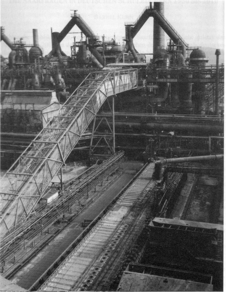
Abb. 6: Koksschrägaufzug zur Gichtbühne
