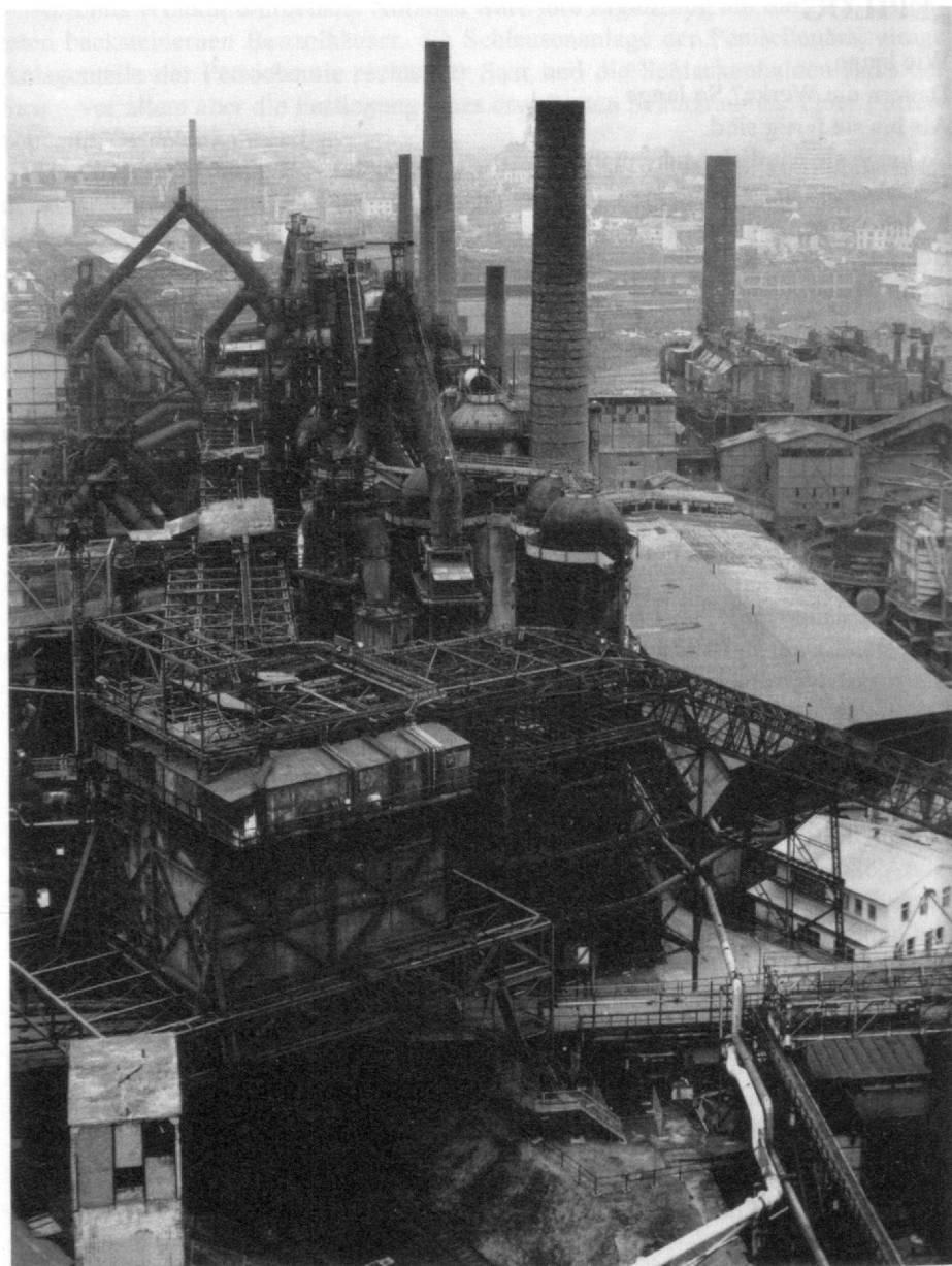
Abb. 1: Alte Völklinger Hütte. Die Silhouette der Hochofengruppe bestimmt sich aus dem Auf- und Absteigen der Gichtglasleitungen, der Kuppeln und Schornsteine der Winderhitzer (Cowper).
