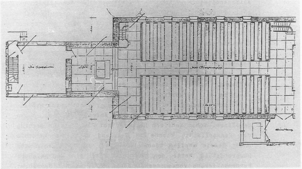
Abb. 23 Saarbrücken-Jägersfreude, evang. Kirche: Grundriß. (aus: M. Malburg 1993)
