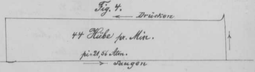
Fig. 4, 5 & 6 Pumpendiagramme einer unterirdischen Compound-Wasserhaltungsmaschine. Druckhöhe 215 m. 1-1,5 atm. pr. Min.
