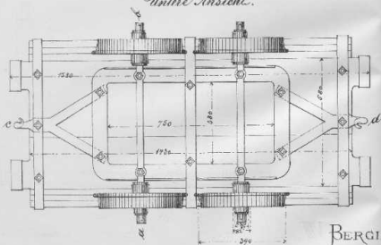
Untere Ansicht.
