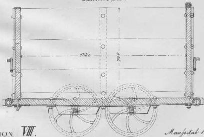
Schnitt cd.
