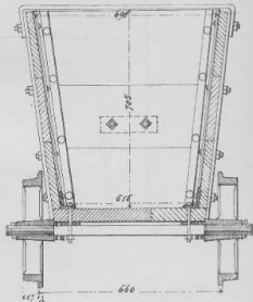
Schnitt cd.
