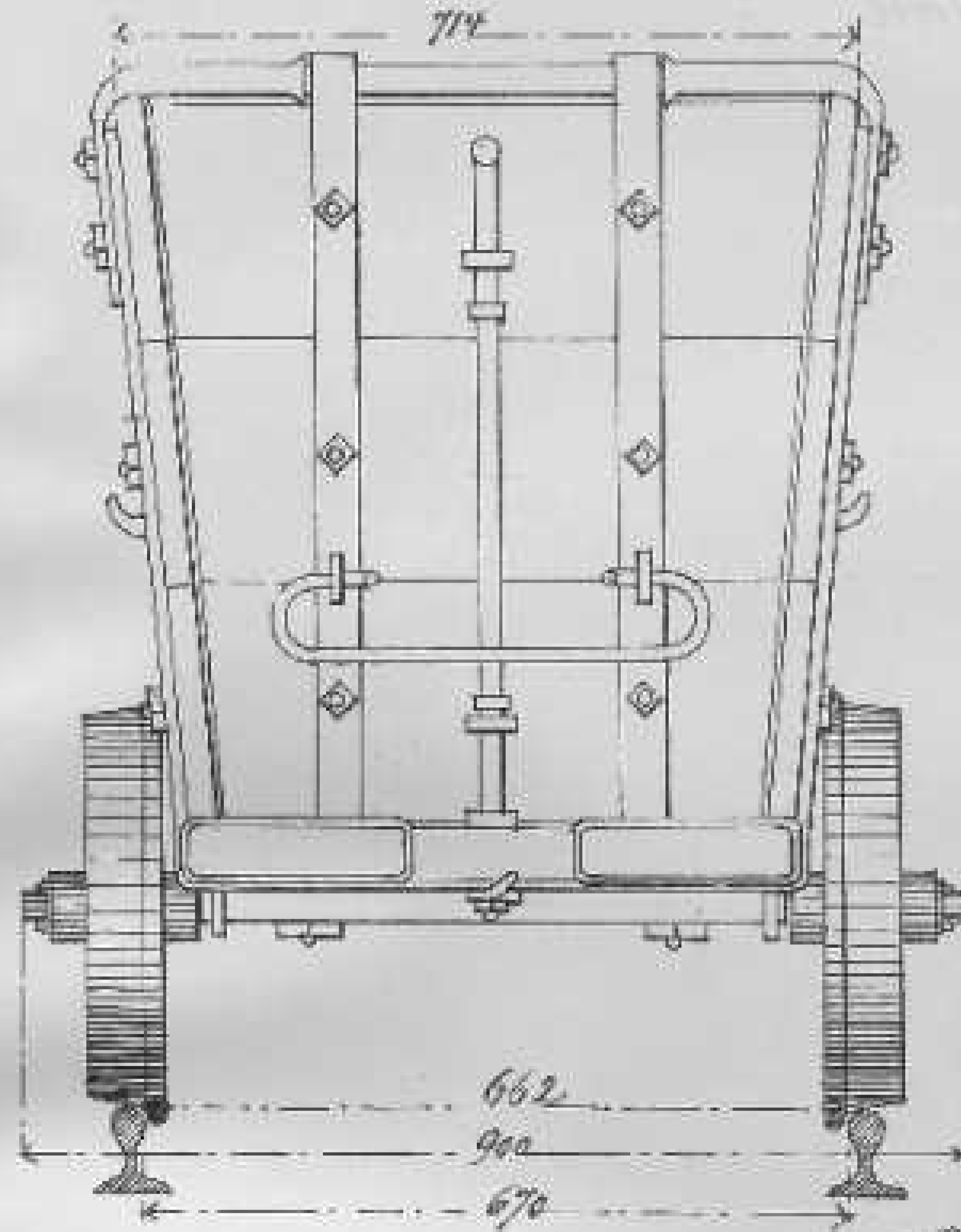
Stirn Ansicht
