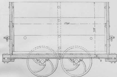
Schnitt cd.
