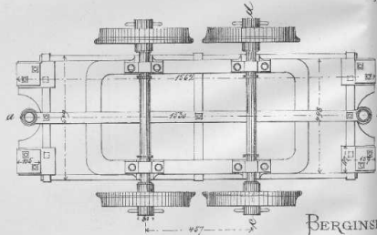
Untere Ansicht.
