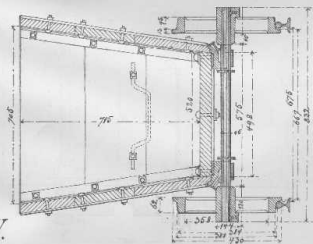
Schnitt cd.
